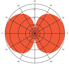
E-plane: 136 MHz
