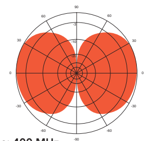
E-plane: 400 MHz
