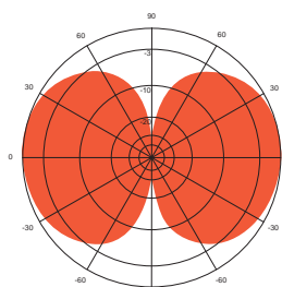
E-plane: 100 MHz
