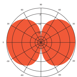
E-plane: 450 MHz
